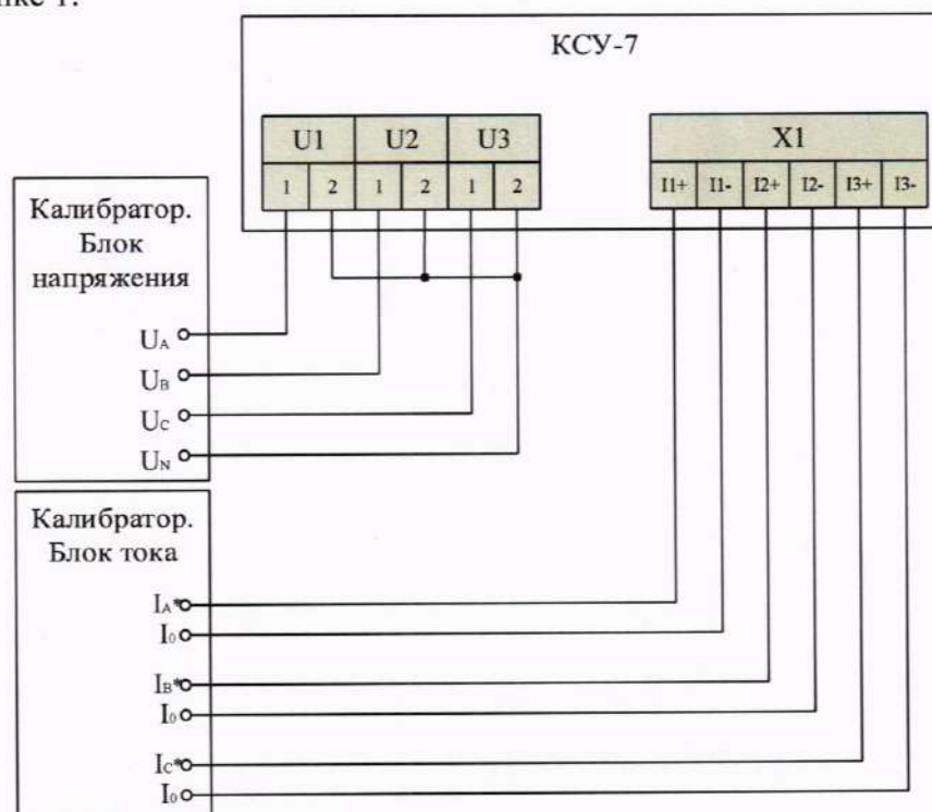
Рисунок 1 – Схема подключения контроллера при определении метрологических характеристик
