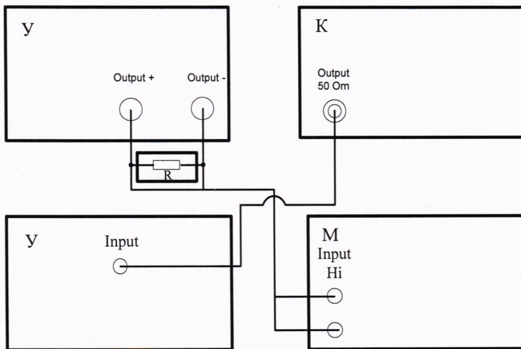
Рисунок 1 - Схема измерений погрешности установки выходного напряжения где:
