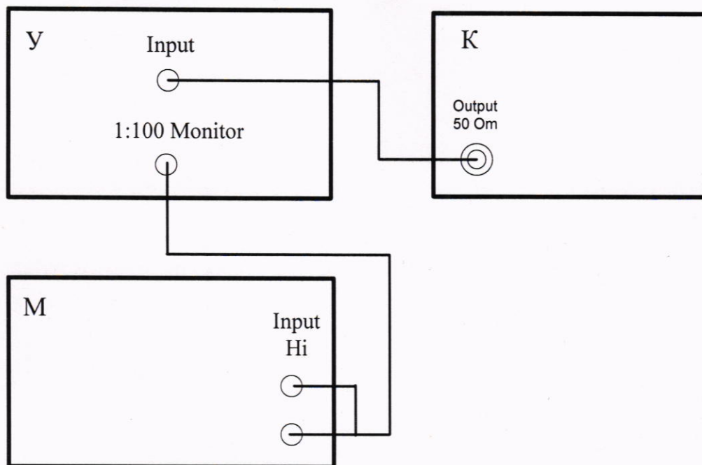
Рисунок 2 – Схема измерений погрешности мониторинга выходного напряжения
