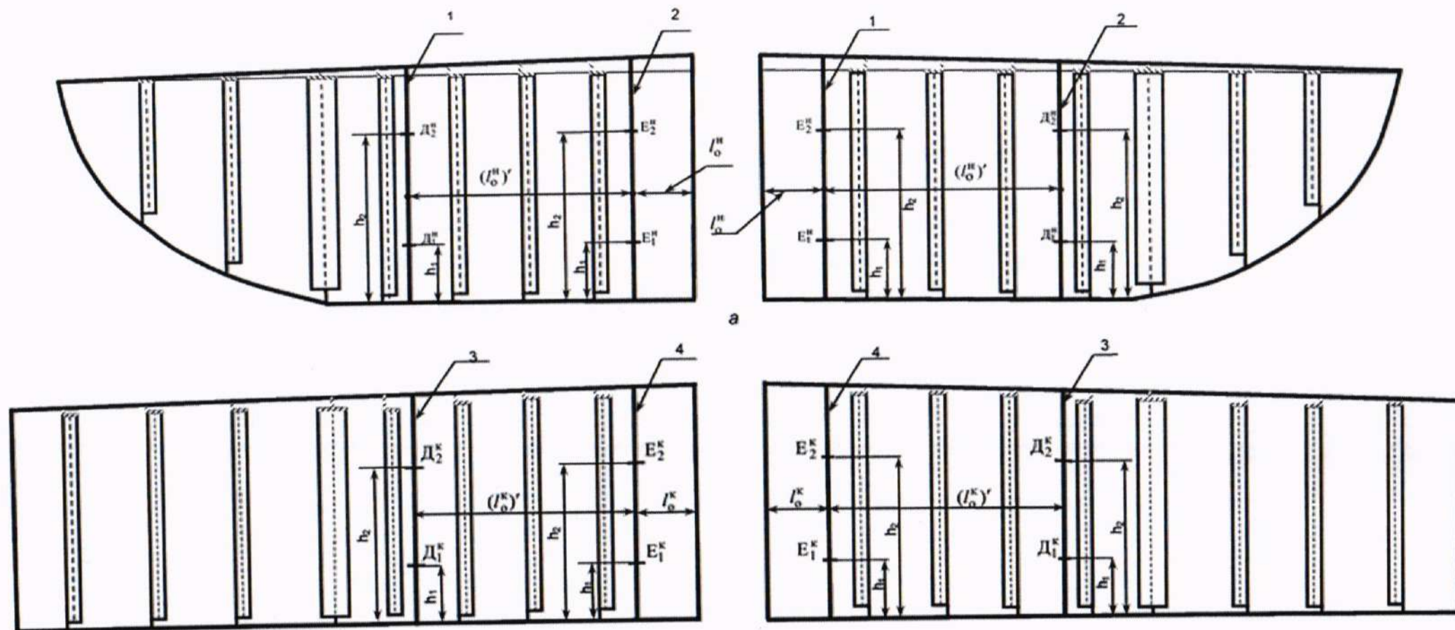
а – носовая поперечная переборка левого и правого бортов; б – кормовая поперечная переборка левого и правого бортов; 1, 2, 3, 4 – вертикальные линии; D_1^H , D_1^K , E_1^H , E_1^K , E_2^H , E_2^K , D_2^H , D_2^K – точки на вертикальных линиях; L_0^H , L_0^K – расстояния от продольной переборки до линий 1 и 4; (L_0^H)' , (L_0^K)' – расстояния между линиями 1, 2 и 3, 4; h_1 – высота точек D_1 и E_1 ; h_2 – высота D_2 и E_2 .
