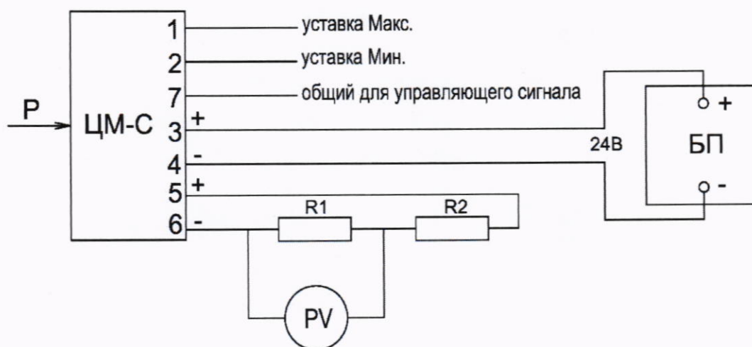
Подключение манометра ЦМ-С с релейным сигнальным устройством
