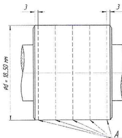
Рисунок 3 – Расположение поперечных сечений роликов (А) диаметром от 18 до 50 мм
