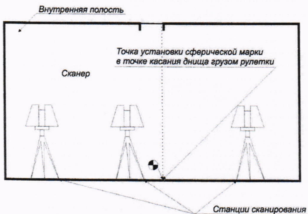
Рисунок А.2 – Схема сканирования внутренней полости резервуара
