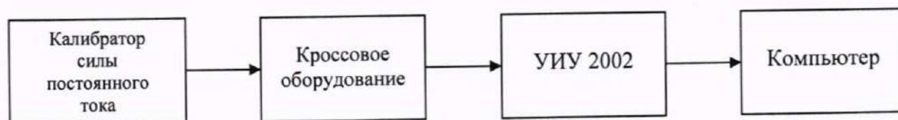
Рисунок 10 - Схема определения метрологических характеристик ИК силы постоянного тока, соответствующей значениям параметра
