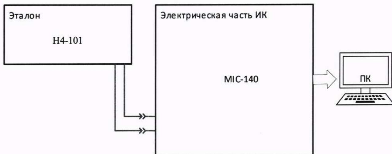
Рисунок 18 – Схема поверки напряжения постоянного тока, соответствующего температуре
