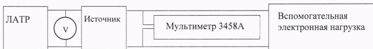
Рисунок 4 - Структурная схема определения нестабильности выходного напряжения постоянного тока, вызванной изменением напряжения питания
