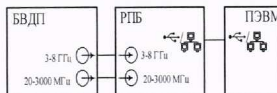
Рисунок 1а – Схема проверки работоспособности для модификаций НАЛС.464344.062, НАЛС.464344.062-02, НАЛС.464344.062-04, НАЛС.464344.062-06
