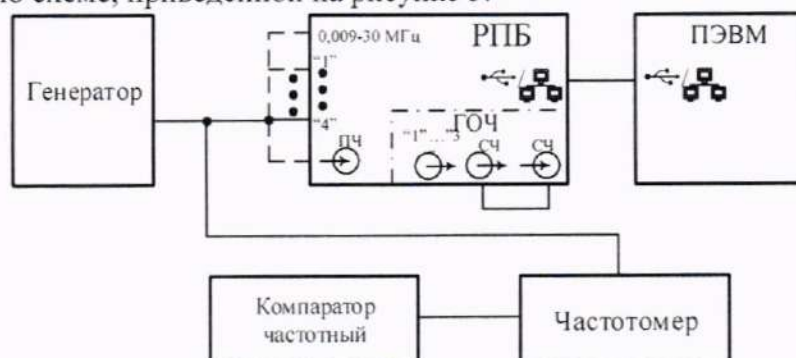
Рисунок 5 – Схема измерений частоты синусоидального сигнала
