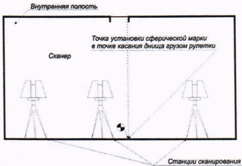
Рисунок А. 1 - Схема измерения базовой высоты резервуара и эталонного расстояния уровнемера
