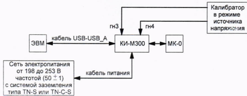
Рисунок 4 – Схема подключения калибратора «Uac»
