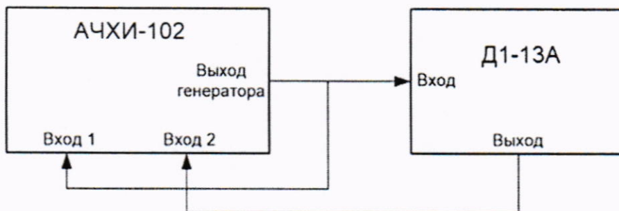
Рисунок 2 – Схема измерения ослабления в диапазоне от 0 до –80 дБ
