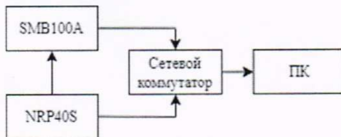
Рисунок 3 – Схема для проведения калибровки подводимой мощности
