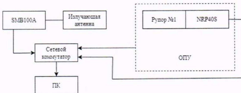
Рисунок 4 – Схема соединений для измерения КУ
