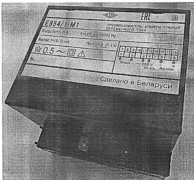
Рисунок 1 – Общий вид и маркировка ИП E854/1-M1 для нужд народного хозяйства
