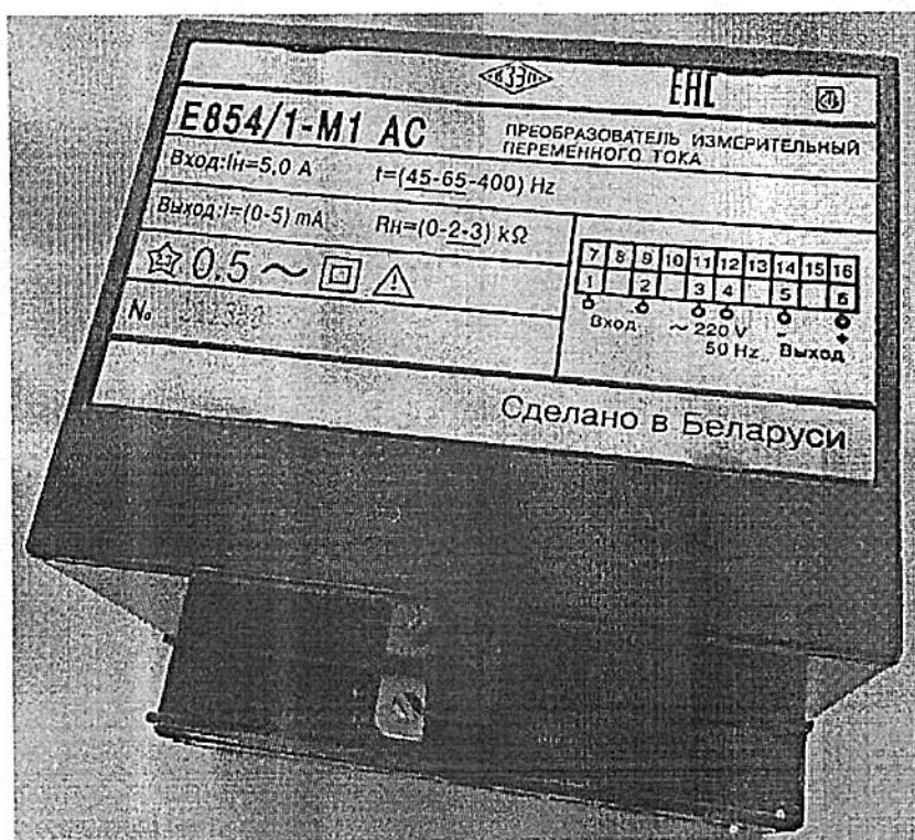
Рисунок 2 – Общий вид и маркировка ИП E854/1-M1 AC для поставки на атомные станции
