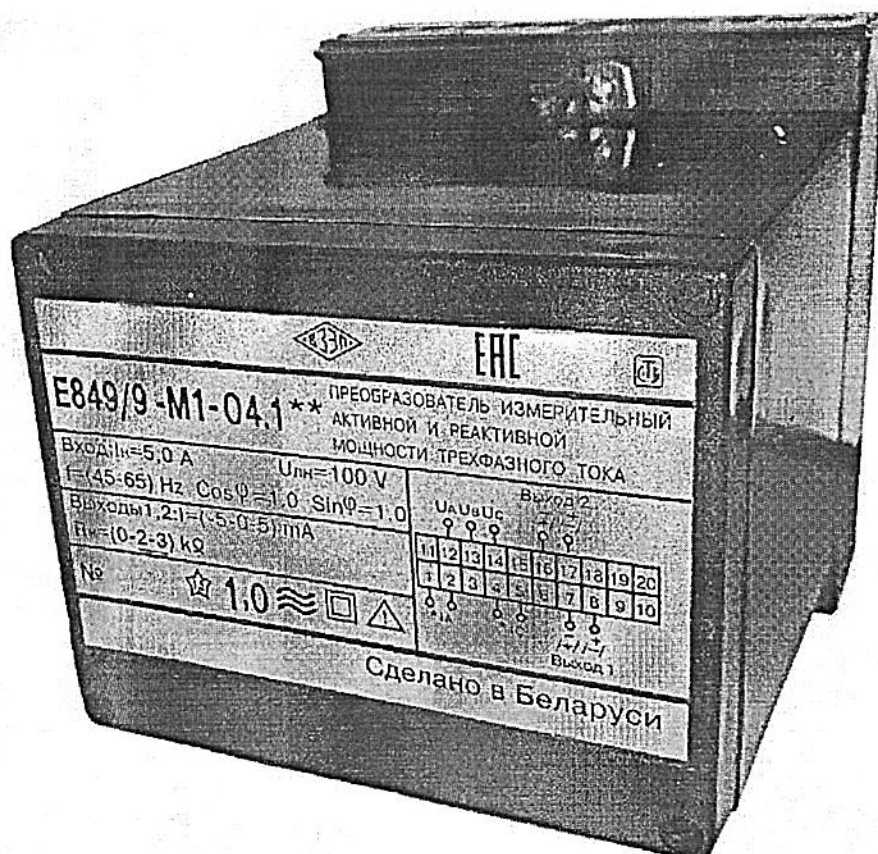
Рисунок 2 – Общий вид и маркировка ИП Е849/9-М1-04.1** для поставки на экспорт (исполнение 04.1**)
