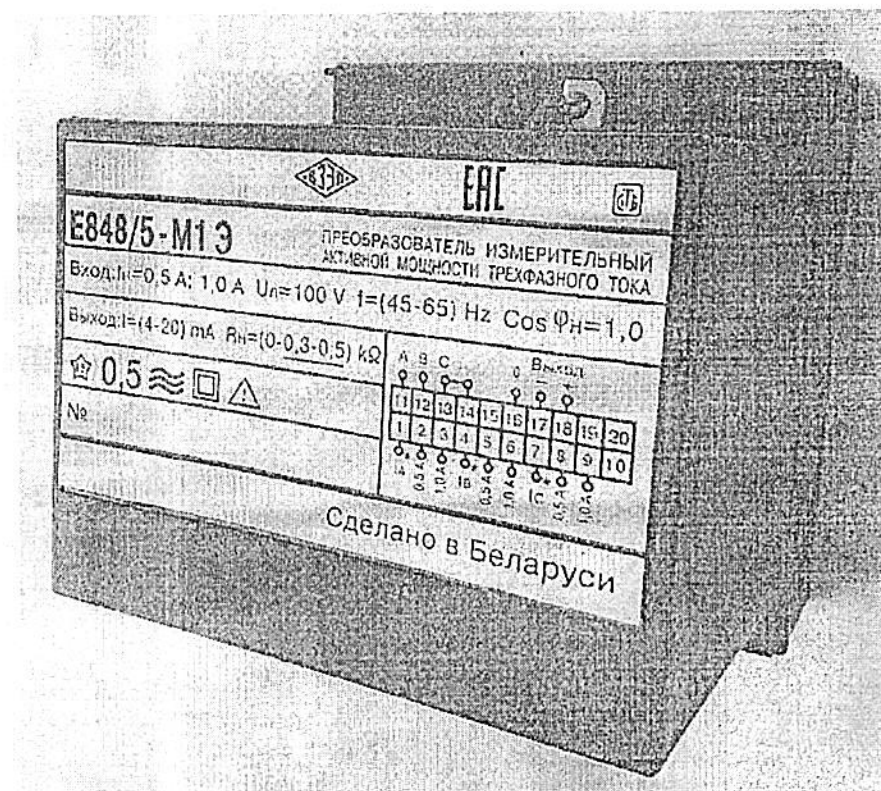
Рисунок 3 — Общий вид и маркировка ИП E848/5-M1 Э для поставки на экспорт в страны с умеренным климатом (экспортное исполнение Э)
