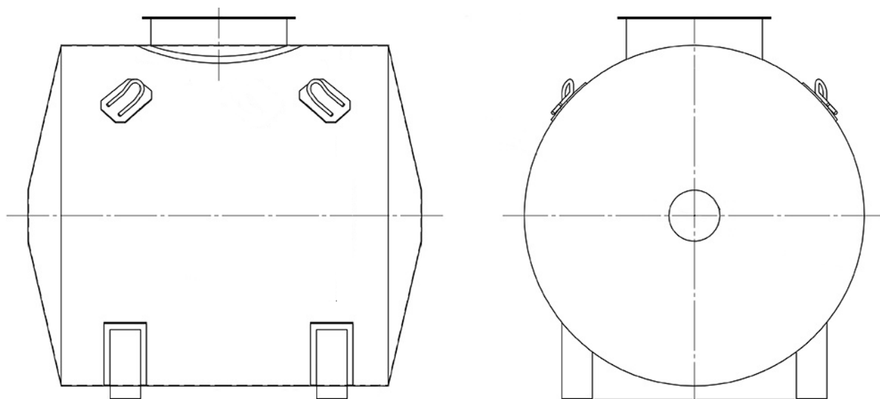
Рисунок 3 – Общий вид резервуара РГСН-5
