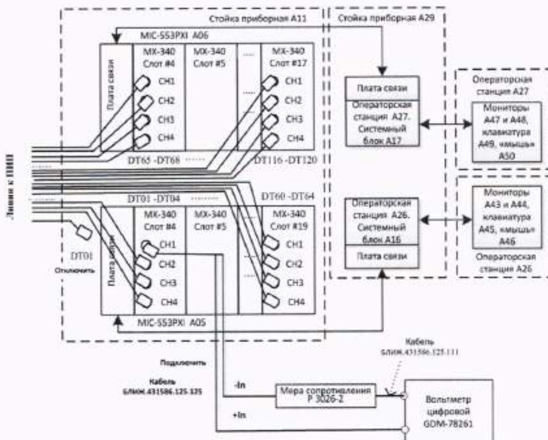
Рисунок 21 - Поверка ИК величины отклонения сопротивления тензорезистора. Схема для поверки электрической части ИК, обеспечивающей подачу тока питания на тензорезистор
