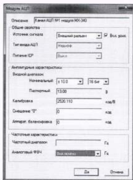
Рисунок 24 – Окно настройки АЦП канала модуля MX-340 для поверки ИК напряжения на измерительной диагонали тензометрического моста
