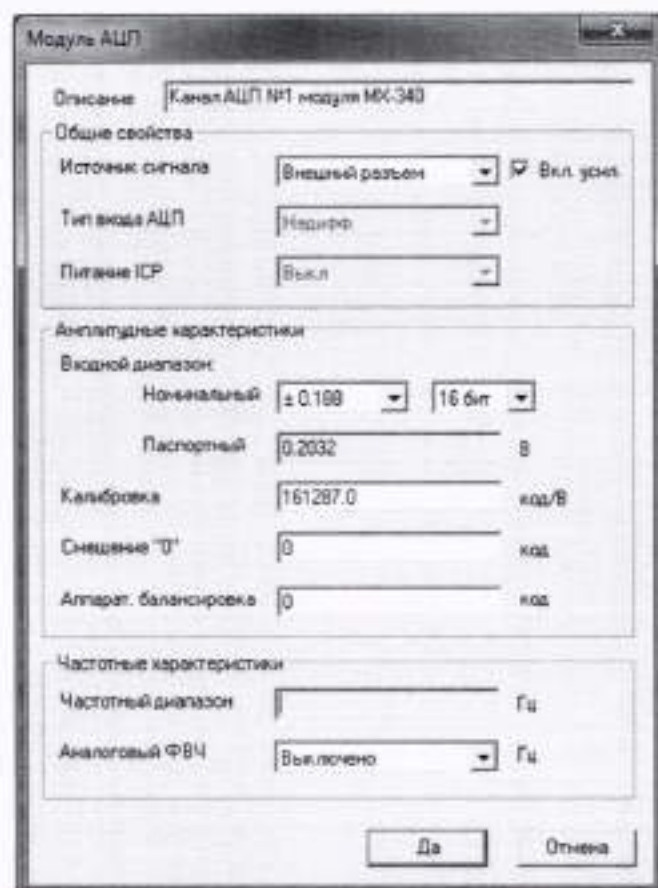
Рисунок 18 – Окно настройки АЦП канала модуля MX-340
