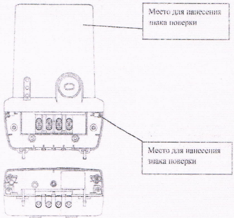
Рисунок 2.4 - Схема (рисунок) с указанием места для нанесения знака поверки на счетчик CE208BY C1
