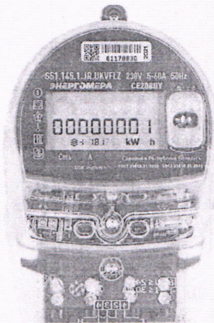
а) общий вид счетчика CE208BY с типом корпуса S7
