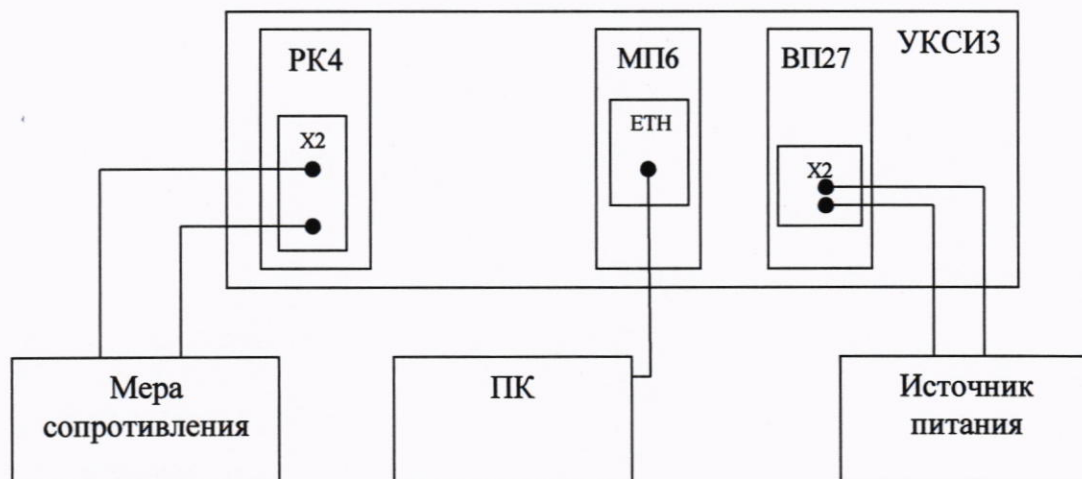
Рисунок 4 - Структурная схема соединения приборов
