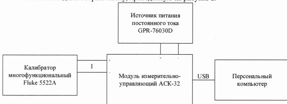
Рисунок 2 – схема определения приведенной (к верхнему пределу измерений) погрешности измерений силы постоянного тока
