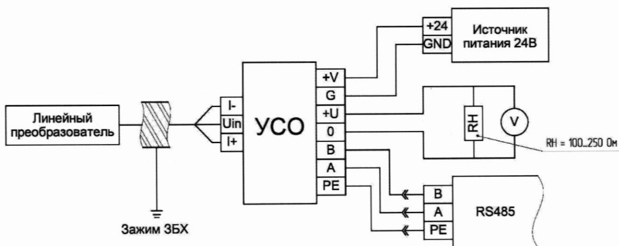
Рисунок Б-2 – Схема подключения датчика при использовании цифрового выхода
