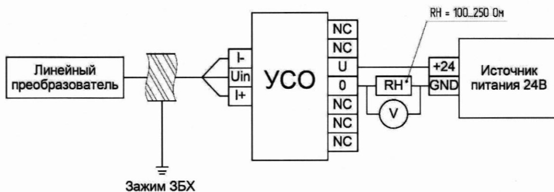
Рисунок Б-1 – Схема подключения датчика при использовании аналогового выхода
