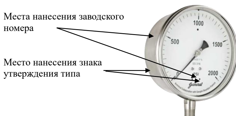
Рисунок 3 – Места нанесения знака утверждения типа и заводского номера
