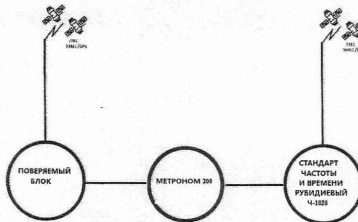
Рисунок 1 – Схема измерений смещения внутренней шкалы времени относительно национальной шкалы времени
