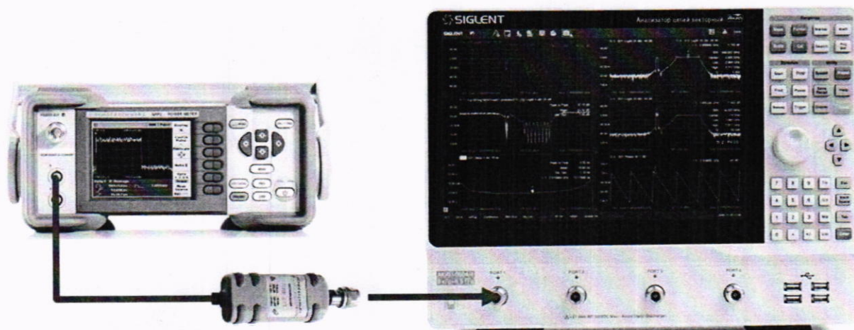
Рисунок 2 – Схема соединения приборов для определения диапазона установки уровня выходной мощности и абсолютной погрешности установки уровня мощности
