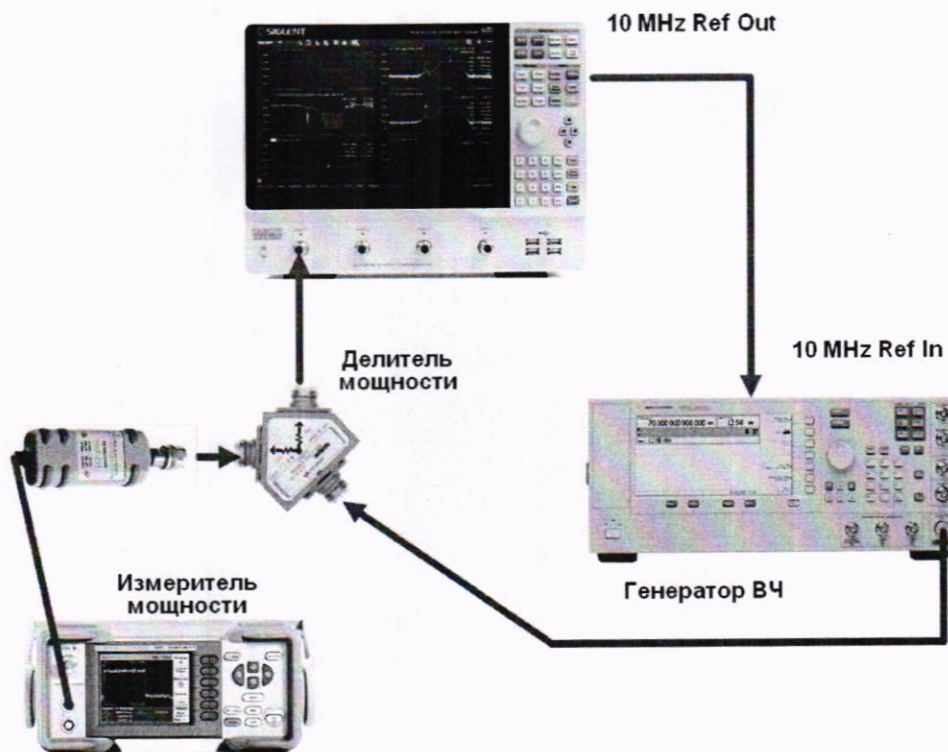
Рисунок 3 – Схема соединения приборов для определения абсолютной погрешности измерений уровня мощности
