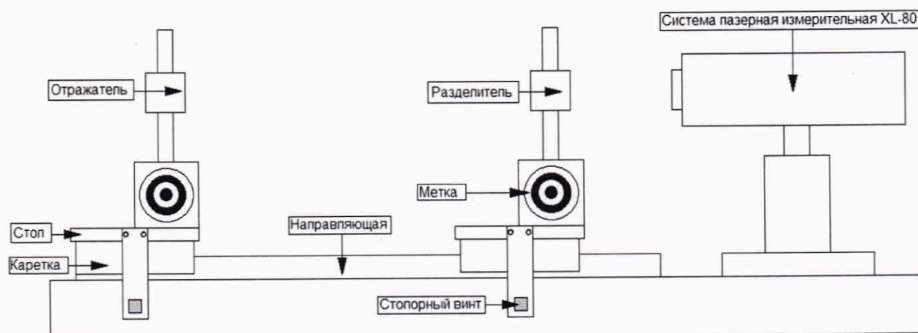
Рисунок 1 – Внешний вид устройства с установленным на нем XL-80 и мишенью
