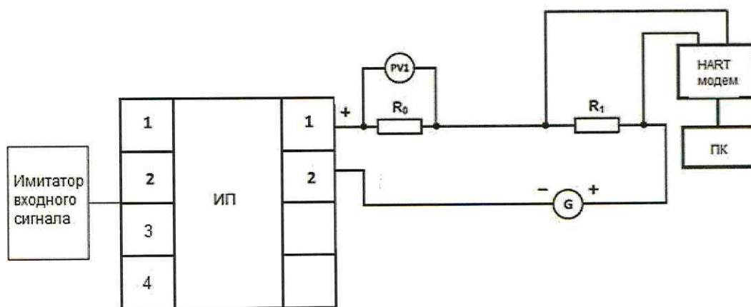
Рисунок А.1 – Схема проверки преобразователя с прямым измерением токового сигнала и подключением HART-модема
