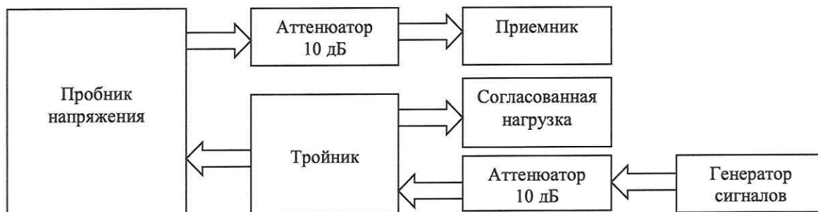
Рисунок 2 - Схема измерений выходного уровня пробника напряжения
