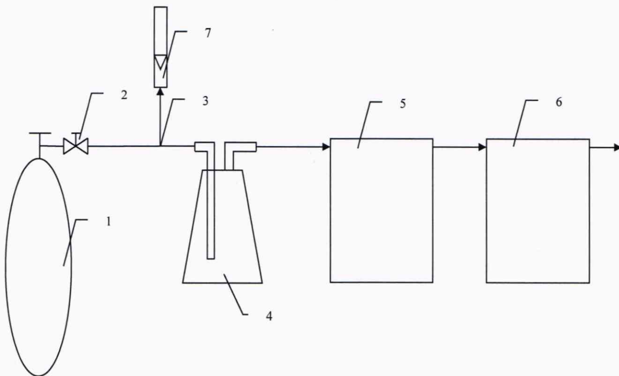
Рисунок В. 1 – Схема подачи аэрозолей
