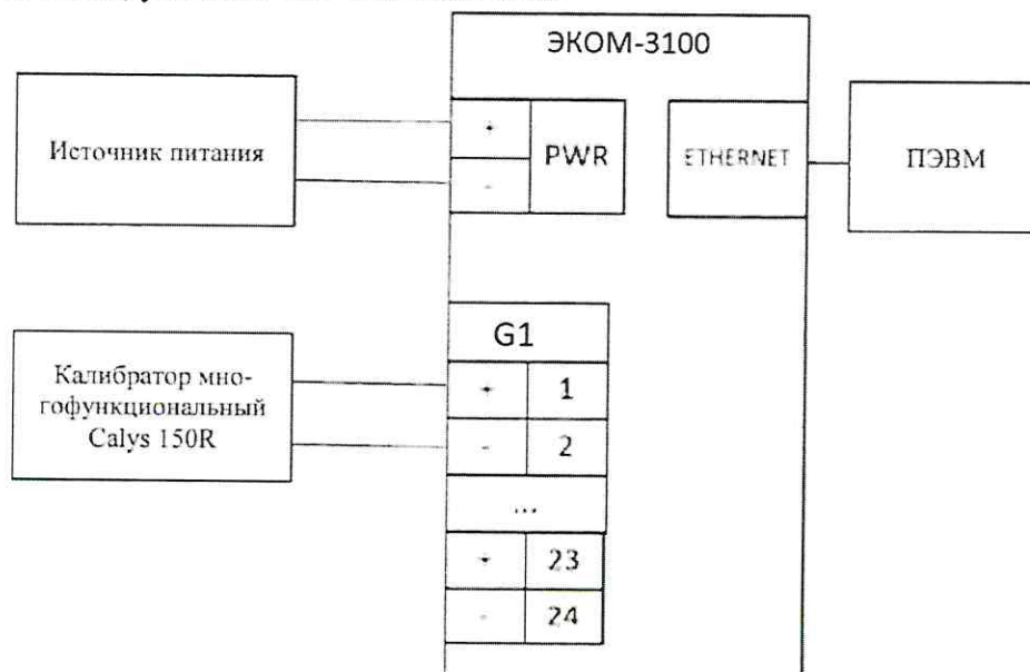
Рисунок 5 – Схема соединений для определения приведенной погрешности измерения постоянных токов
