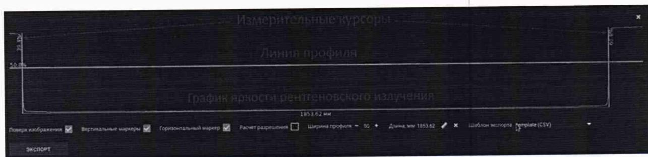
Рисунок 2 – График яркости рентгеновского излучения
