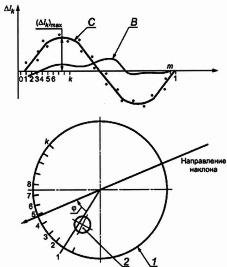
1 - контур днища резервуара; 2 - измерительный люк; \Delta l_k - функция, вычисляемая по формулам (4) и (5); C, B - графики функции \Delta l_k при наличии и отсутствии наклона резервуара соответственно; (\Delta l_k)_{\max} - максимум функции \Delta l_k ; m - число разбинок; k - номер разбишки; \varphi - угол направления наклона резервуара
