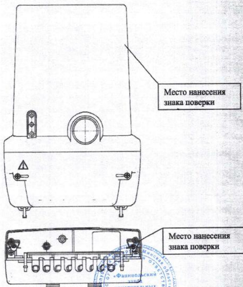
Рисунок 2.6 - Схема (рисунок) с указанием места для нанесения знаков поверки на счетчик CE318BY S3
