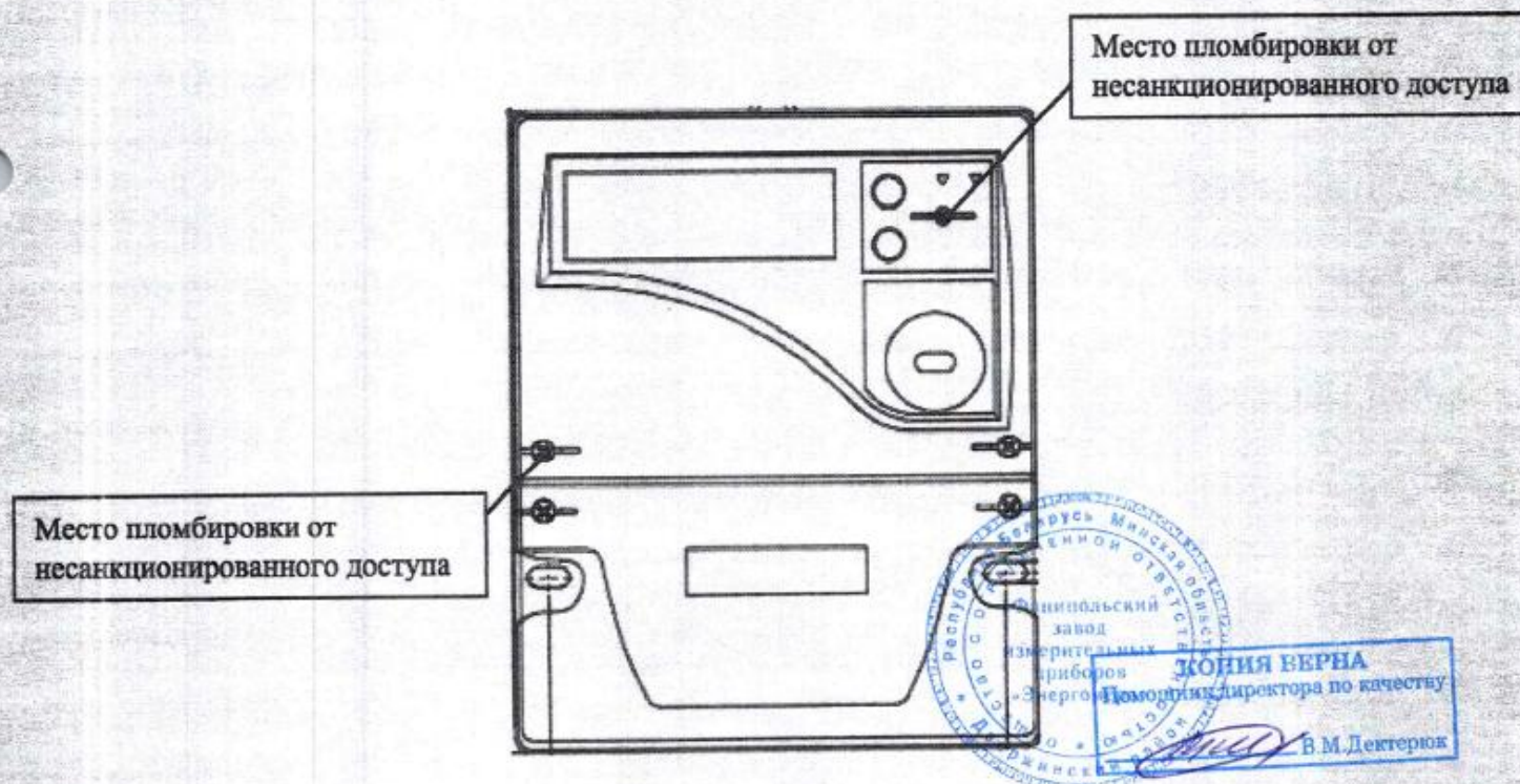
Рисунок 3.2 - Схема (рисунок) с указанием мест пломбировки от несанкционированного доступа на счетчик СЕ318BY S31
