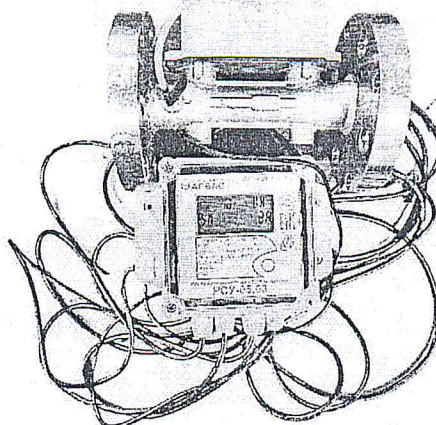
в) Расходомеры-счетчики ультразвуковые модификаций PCY-05.03 IP68 раздельного исполнения
