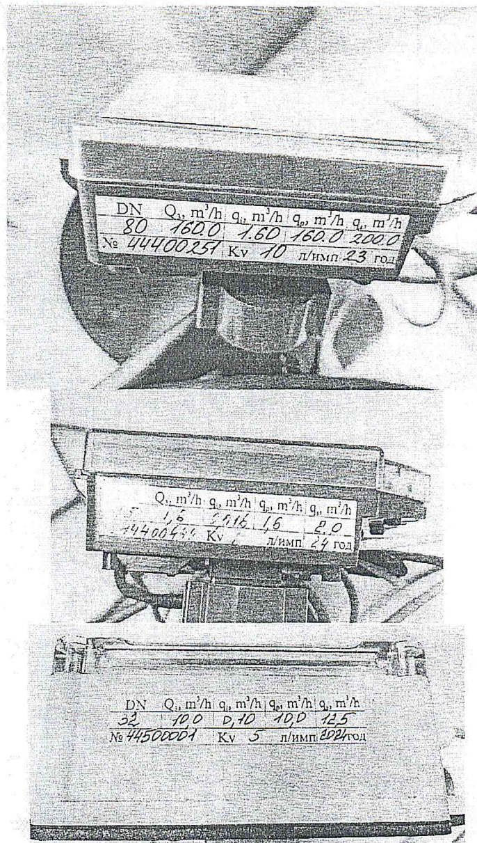
Рисунок 1.2 — Фотографии маркировки расходомеров-счетчиков ультразвуковых РСУ-05 (изображение носит иллюстративный характер)
