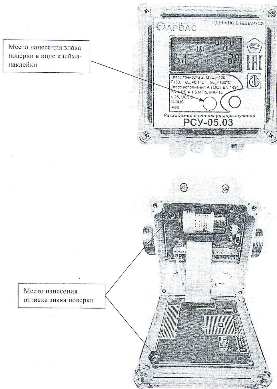
Рисунок 2.2 – Схема (рисунок) с указанием места для нанесения знака поверки для расходомеров-счетчиков ультразвуковых PCSU-05 со степенью защиты оболочки IP68
