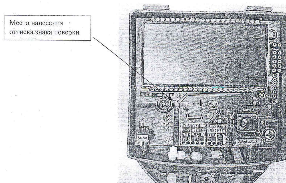
Рисунок 2.1 – Схема (рисунок) с указанием места для нанесения знака поверки для расходомеров-счетчиков ультразвуковых PCSU-05 со степенью защиты оболочки IP54
