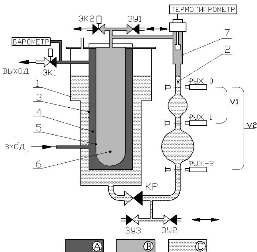
Рисунок 2 - Конструктивная схема мерного блока устройства расходомерного УР-1.0
