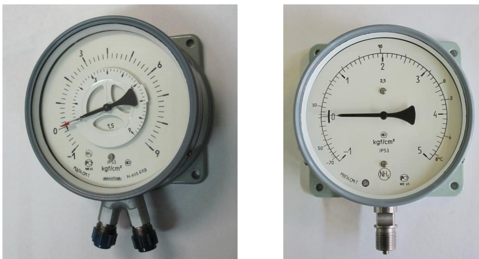
Рисунок 1 - Фотографии общего вида приборов
