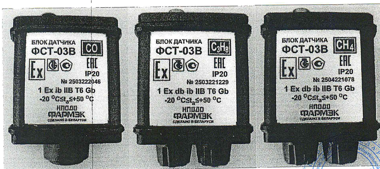
Рисунок 1.3 – Фотографии общего вида и маркировки блоков датчиков газоанализаторов ФСТ-03В (изображение носит иллюстративный характер)
