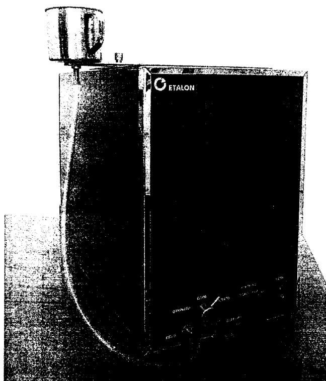
Рисунок 1. Внешний вид и маркировка калориметра сжигания с бомбой (жидкостные) В-08МА «К».
